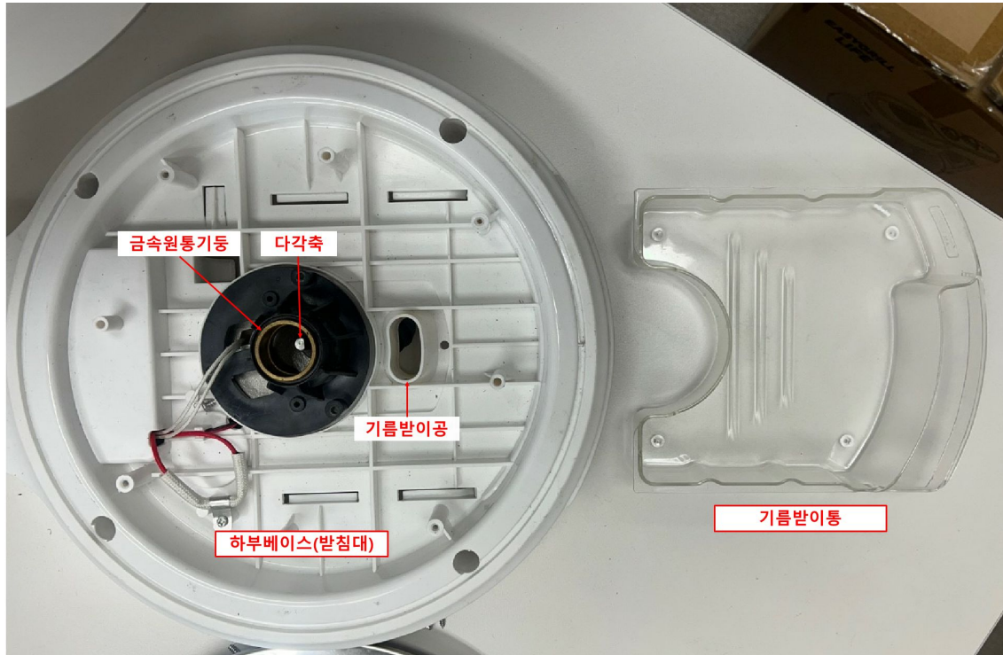
하부베이스(받침대) 구성
